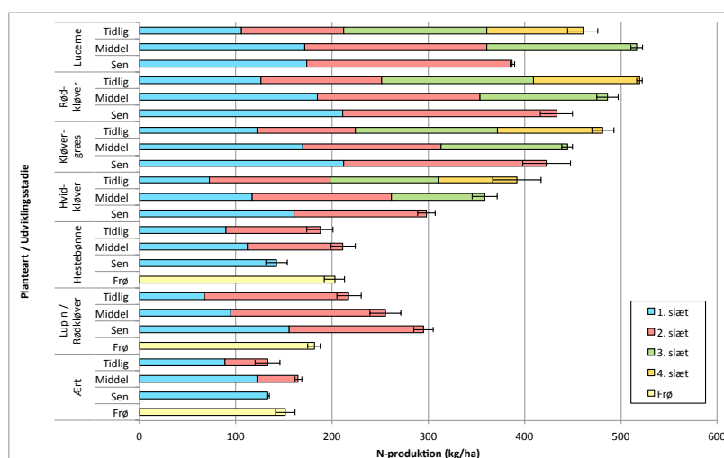
Figur 1. Produktion af kvælstof med bælgplanter høstet og genhøstet på forskellige udviklingsstadier i Årslev.
